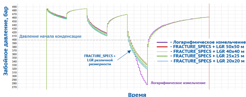
Рис. 10. Динамика забойного давления при моделировании работы скважины на трех режимах при разном измельчении ячейки с использованием виртуальных перфораций
