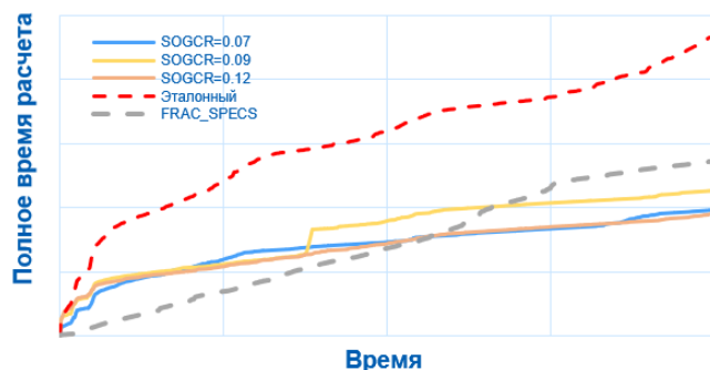
Рис. 13. Полное время расчета ГДМ при разных уровнях измельчения ячейки с трещиной ГРП
