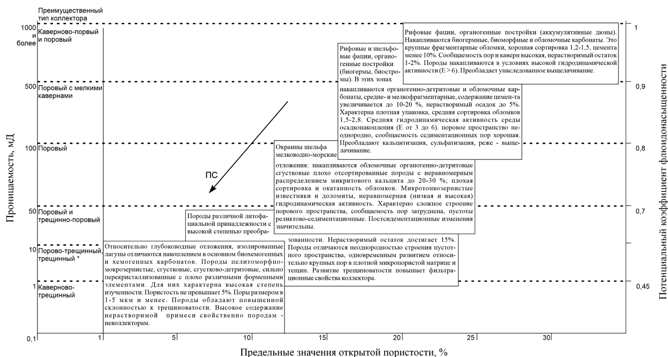
Рис. 5. Принципиальная схема формирования карбонатных пород коллекторов в породах различной литофациальной принадлежности (Багринцева, 1999)
