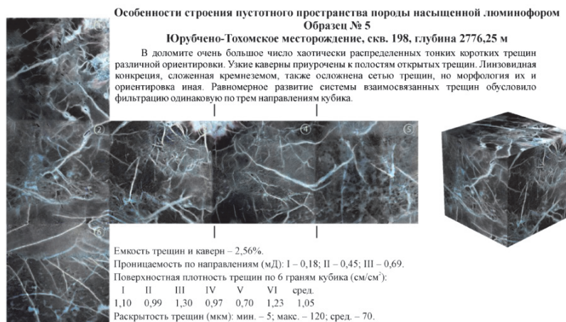
Рис. 2. Особенности строения пустотного пространства карбонатных пород-коллекторов после обработки пенетрантом и аналитических исследований (Багринцева и др., 2015)
