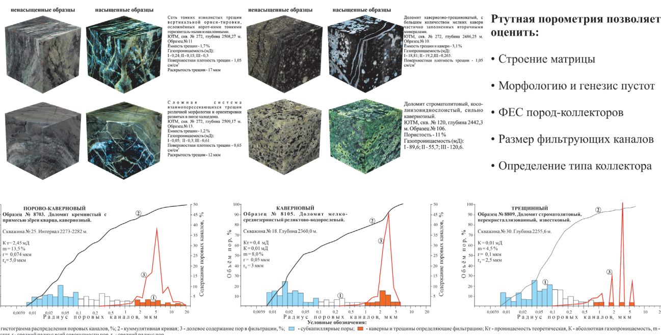
Рис. 6. Ртутная порометрия — определение фильтрующих каналов и типа коллектора (Багринцева и др., 2013)
