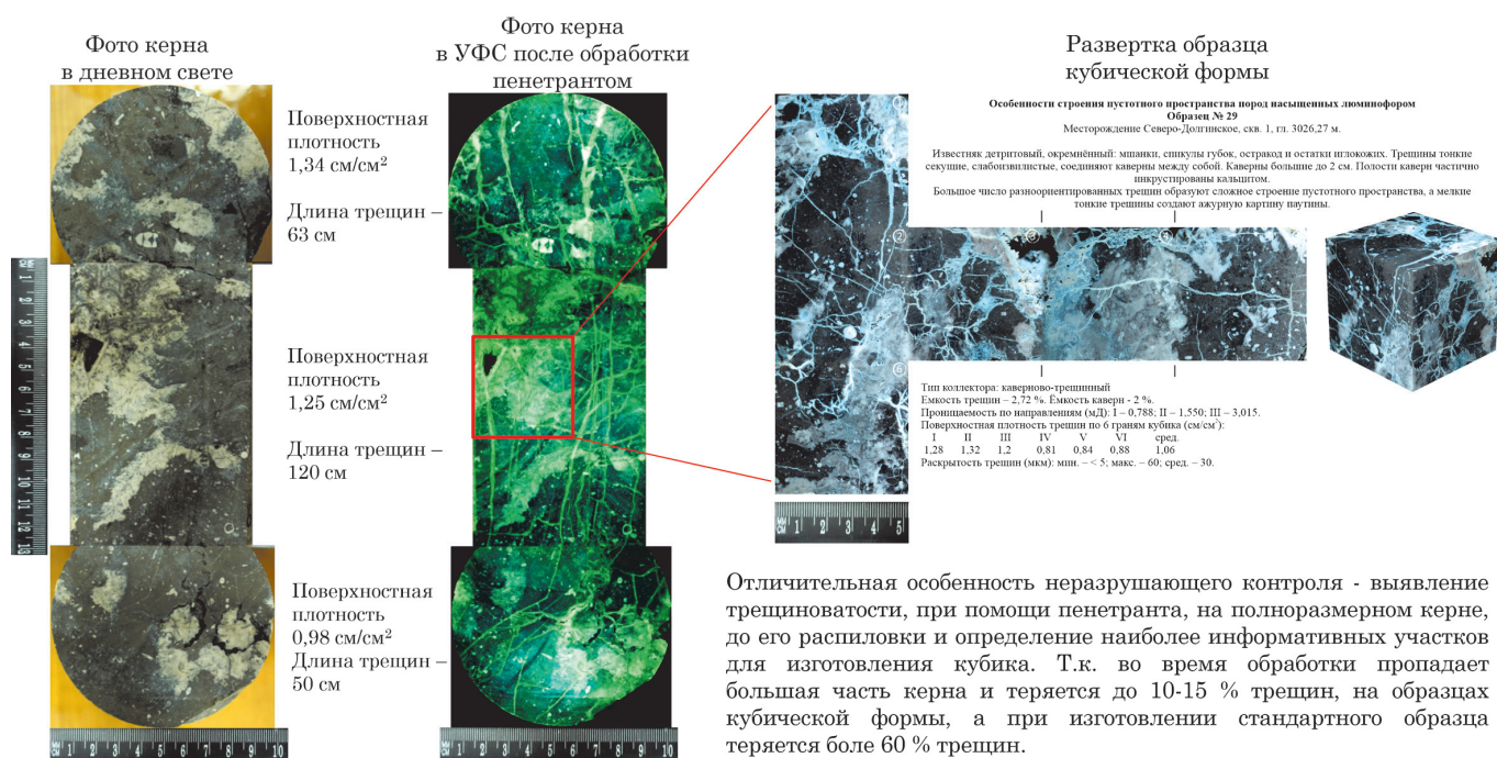
Рис. 3. Исследования трещиноватости и фильтрационно-емкостных свойств методом К.И. Багринцевой (Сауткин и др., 2019)
