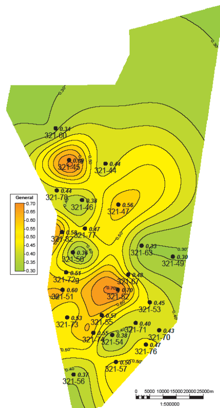
Рис. 5. Схема распространения трещинных коллекторов в талахском горизонте
