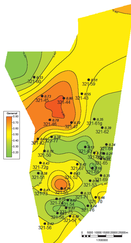
Рис. 4. Схема распространения трещинных коллекторов в хамакинском горизонте
