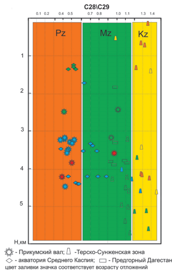
Рис. 3. Ранжирование исследованных нефтей по «геохимическому возрасту» (по биомаркерным показателям)
