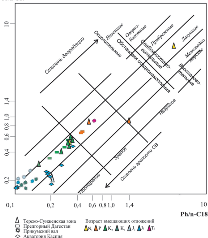
Рис. 2. График Кеннона-Кессоу для исследованных нефтей Предкавказья
