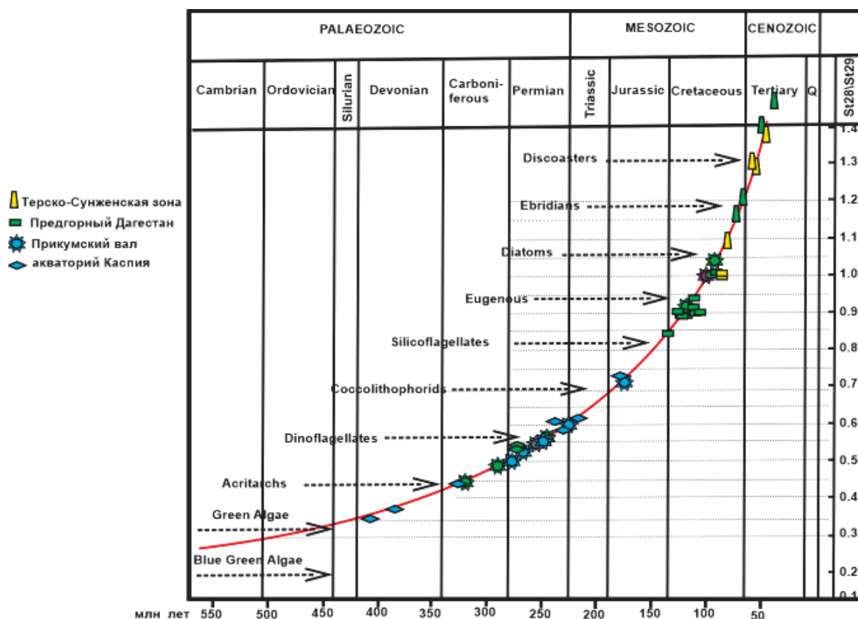
Рис. 4. Распределение нефтей Терско-Каспийского НГБ на адаптированной графике Грэхема (Grantham, Wakefield, 1988) для определения геологического возраста нефтей по соотношению стеранов C28/C29
