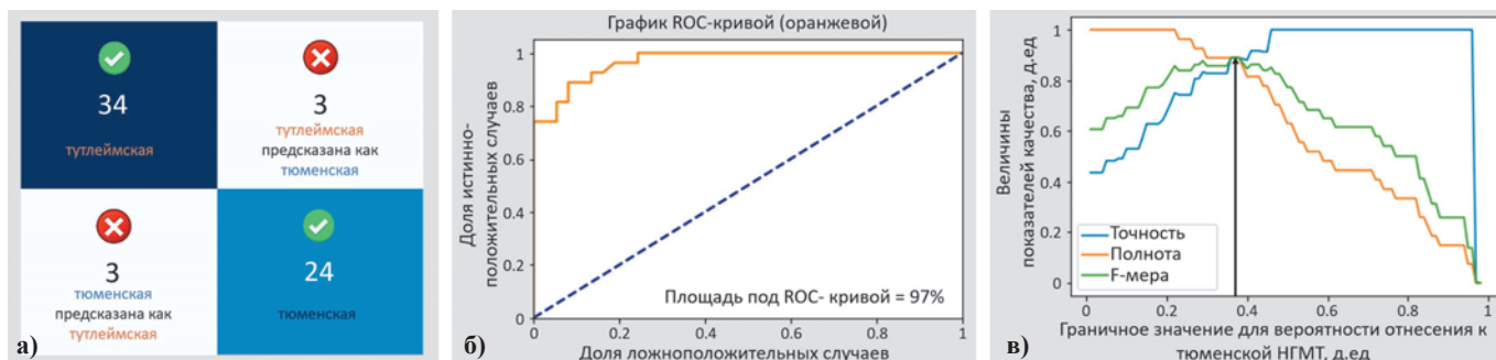
Рис. 8. а) Матрица ошибок, б) ROC-кривая и в) график зависимости F-меры, точности и полноты от граничного значения вероятности отнесения к тюменской НГМТ
