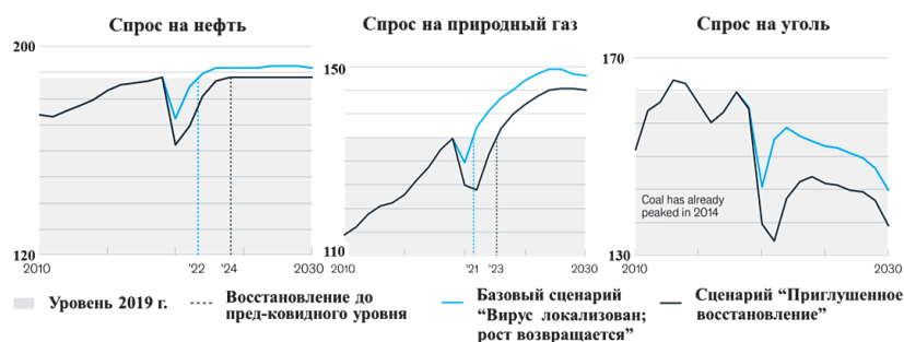
Рис. 6. Глобальный спрос на основные первичные энергоресурсы, млн тераджоулей (million TJ). Источник: (McKinsey Energy Insights..., 2020).
