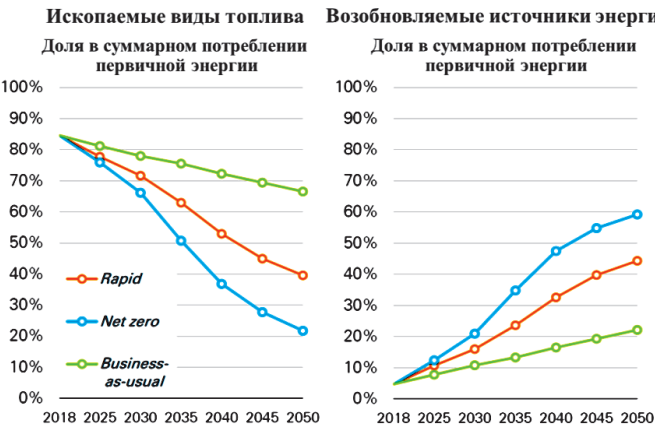
Рис. 10. Доля ископаемых видов топлива и ВИЭ в различных сценариях BP Energy Outlook 2020. * – ВИЭ без учёта крупных ГЭС. Rapid – Сценарий быстрого перехода; Net Zero – Сценарий нулевых выбросов; Business as Usual – Сценарий обычного развития. Источник: (BP Energy Outlook 2020..., 2020).
