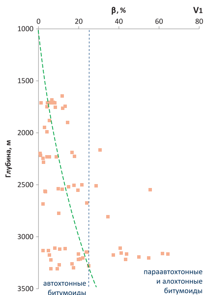
Рис. 4. Зависимость изменения битумоидного коэффициента с глубиной проб нижневендского венда
