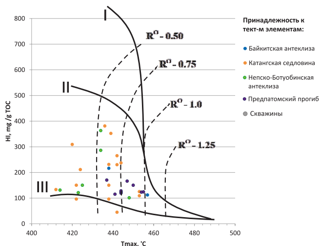
Рис. 8. Диаграмма с соотношением параметров HI-Tmax образцов нижневендских НГМТ
