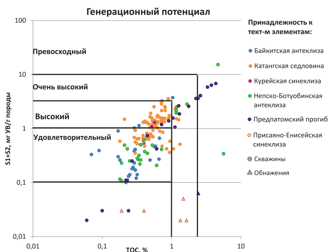
Рис. 6. Генерационный потенциал нижневендских отложений
