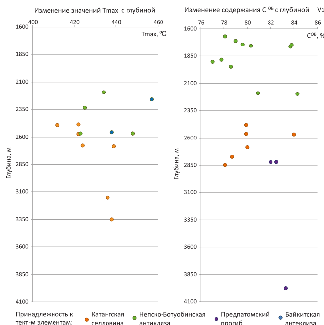
Рис. 12. Изменение показателей C^{OB} (в процентах по оси абсцисс на графике слева) и T_{max} (в м по оси абсцисс на графике справа) с глубиной (в м по оси ординат) образцов НГМТ отложений нижнего венда
