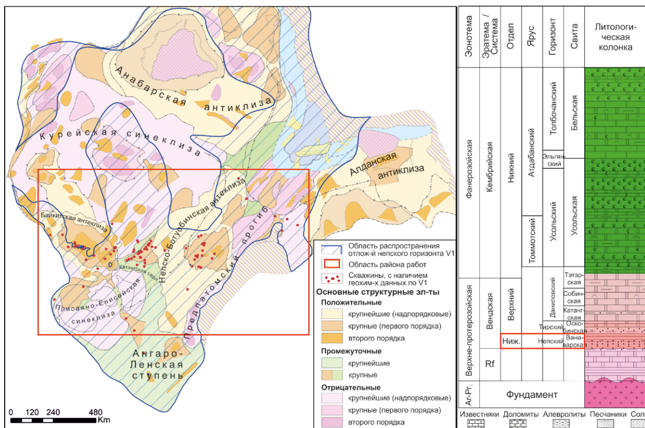
Рис. 1. Структурно-тектоническая карта (Старосельцев и др., 2015, с изменениями) и сводная лито-стратиграфическая колонка с выделением области и интервала исследования
