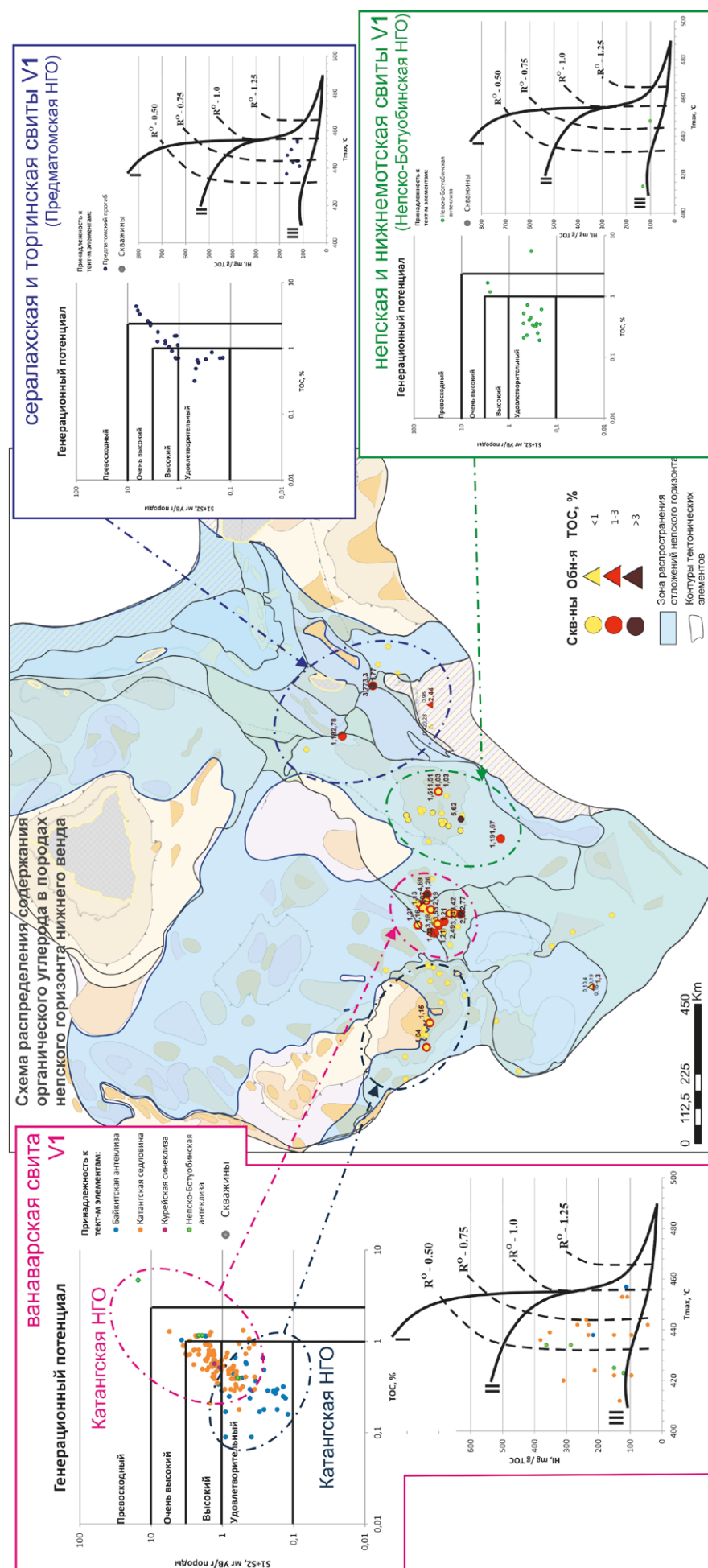
Рис. 7. Схема с распространением точек замеров TOC пород непского нижневендского горизонта из скважин и обнажений
