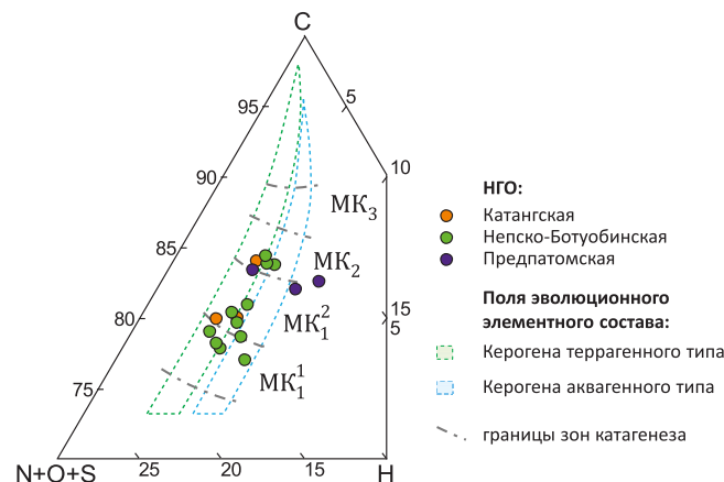
Рис. 10. Тригонограмма элементного состава керогена образцов нижнего венда в %, основанная на модели эволюции элементного состава керогена в катагенезе (Конторович, 1964; Богородская и др., 2005).
