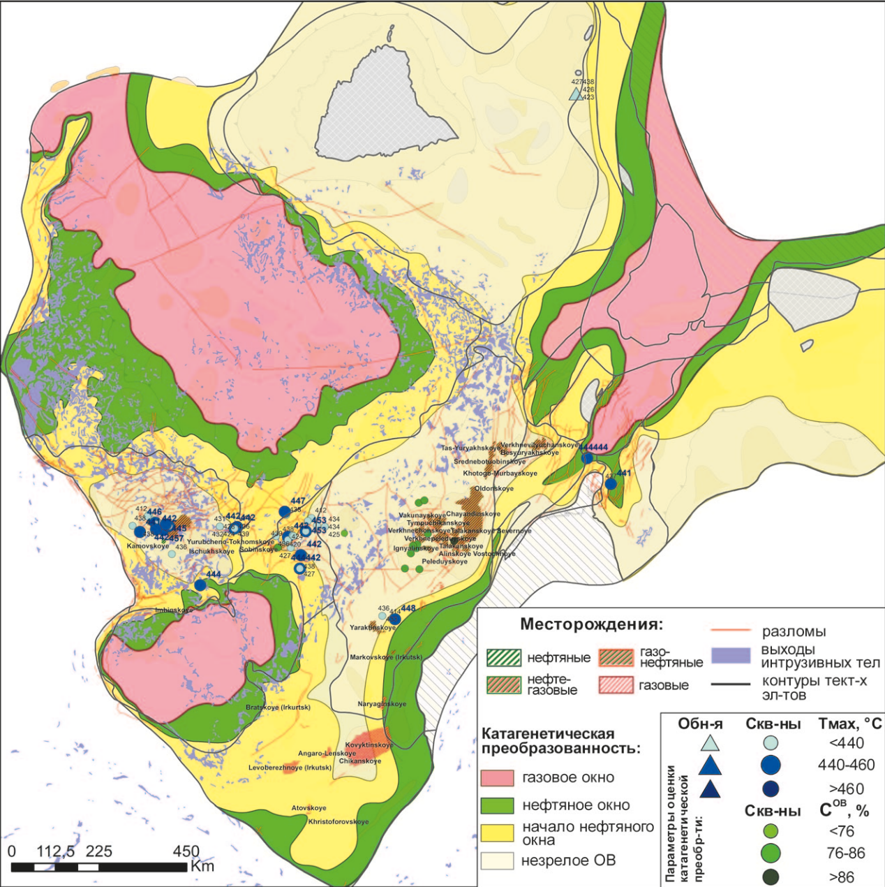
Рис. 11. Схема катагенетической преобразованности ОВ нефтематеринских формаций нижневендского комплекса
