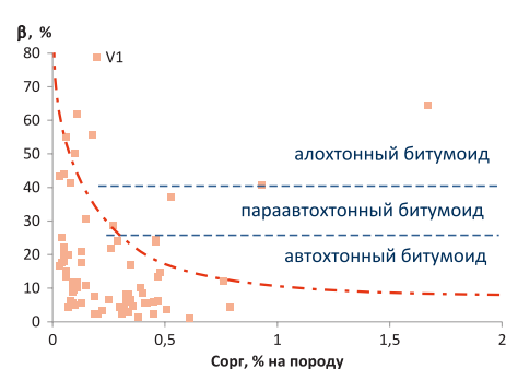
Рис. 3. Зависимость битумоидного коэффициента ( \beta ) от содержания органического углерода в отложениях нижнего венда из скважин и обнажений Восточно-Сибирского НГБ
