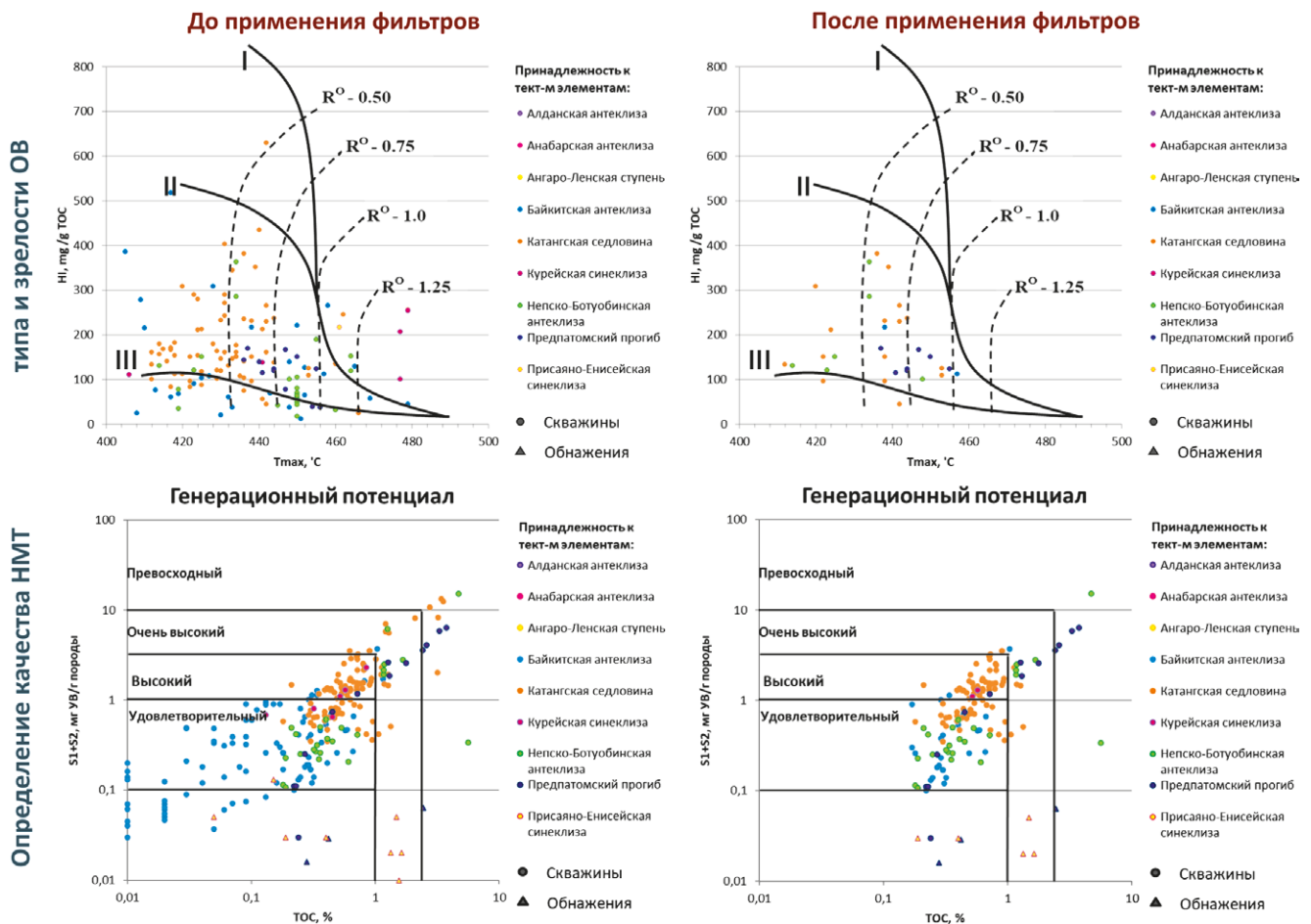
Рис. 5. Сравнение модифицированных диаграмм Ван-Кревелена и графиков оценки генерационного потенциала до и после применения фильтров
