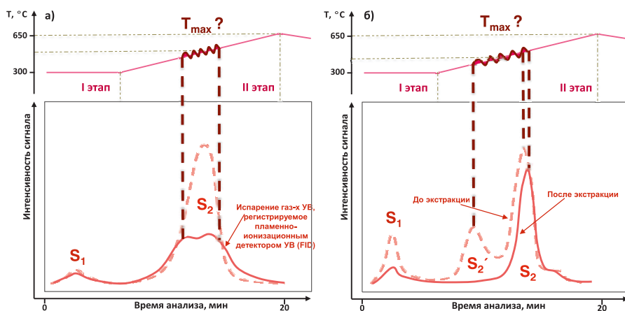
Рис. 2. Примеры пирогрaмм с низким значением S_2 (а) и наличием второго пика S_2' у неэкстрагированного образца (б), отражающие сложность выделения пика выхода УВ и определения времени замера температуры
