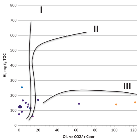
Рис. 9. Диаграмма с соотношением параметров HI-OI образцов нижневендских НГМТ
