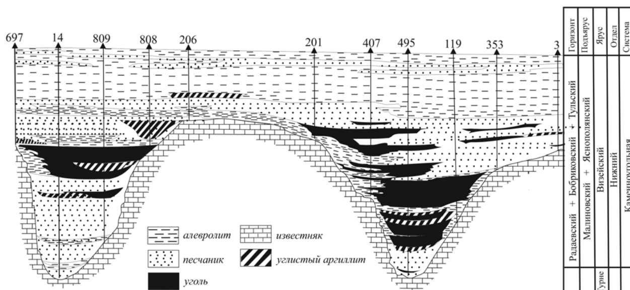
Рис. 1. Палеоврезы в турнейских известняках – вместилище визейских угольных залежей. Угольно-нефтяное месторождение Арлан (Угольная база России, 2000)
