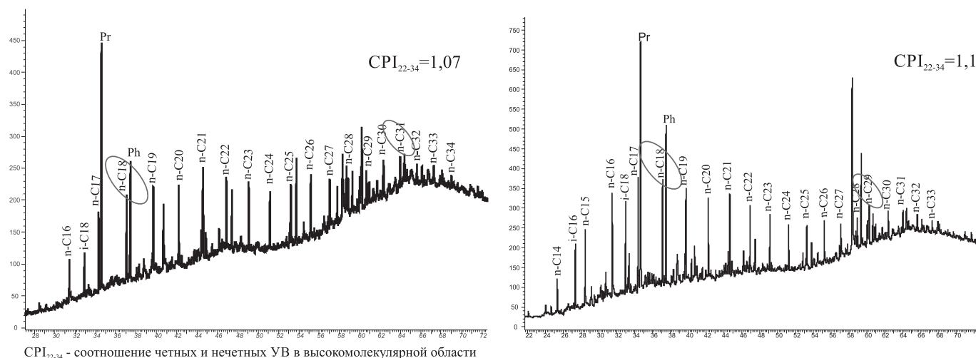
Рис. 2. Хроматограммы алкановых УВ доманикового горизонта (слева – Верхне-Гарейская площадь, известковая глина, справа – Сулимская площадь, микритовый известняк)
