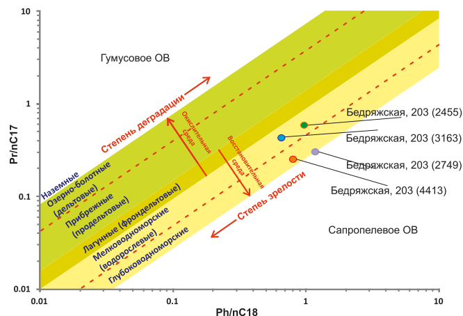
Рис. 5. Диаграмма Кеннона-Кессоу для образцов калтасинской свиты
