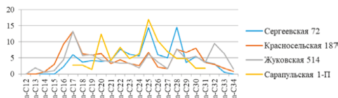
Рис. 11. Графики распределения членов гомологического ряда n -алканов битумоидов верещагинской свиты
