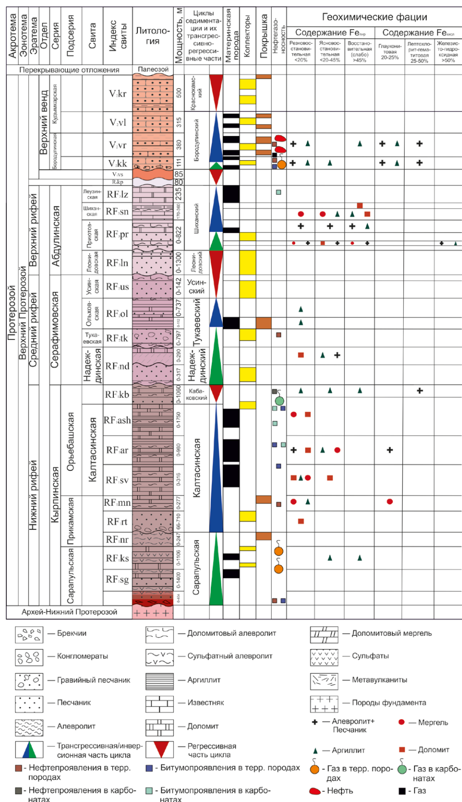
Рис. 2. Сводный литолого-стратиграфический разрез рифей-вендских отложений северной части Камско-Бельского авкогена (на основании данных С.Е. Башковой, О.Б. Дьяконовой, И.С. Хопта). Прим.: названия свит RF_{sg} – сигаевская; RF_{ks} – костинская; RF_{nr} – норкинская; RF_{rt} – ротковская; RF_{mn} – минаевская; RF_{kb} – кабаковская; RF_{nd} – надеждинская; RF_{tk} – тукаевская; RF_{ol} – ольховская; RF_{us} – усинская; RF_{ln} – леонидовская; RF_{pr} – притовская; RF_{sn} – шиханская; RF_{lz} – леузинская; RF_{kr} – кичкаская; V_{vs} – веслянская; V_{kk} – кыквинская; V_{vr} – верещагинская; V_{vl} – велвинская; V_{kr} – краснокамская. Подсвит калтасинской свиты ( RF_{kl} ): RF_{sv} – саузовская; RF_{ar} – арланская; RF_{ash} – ашитская.
