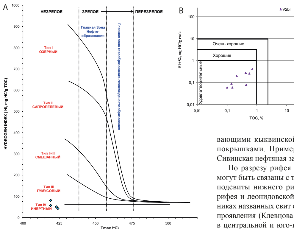
Рис. 9. Пиролитические характеристики пород бородулинской серии: А – модифицированная диаграмма Ван-Кревелена; В – диаграмма генерационного потенциала
