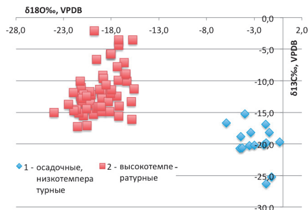
Рис. 4. \delta^{13}\text{C} и \delta^{18}\text{O} двух типов карбонатов, связанных с наложенными процессами
