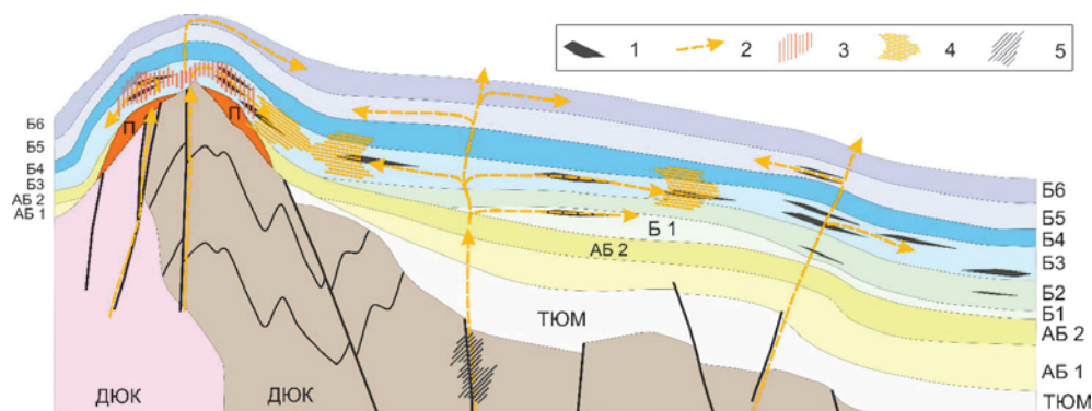
Рис. 9. Принципиальная модель функционирования гидротермальных систем на постседиментационном этапе развития. ДЮК – доюрский комплекс; ПАХ – пахомовская; ТЮМ – тюменская; АБ – абалакская; Б – БВУФ; номерами показаны пакки; 1 – первичные флюидопроницаемые зоны; 2 – гидротермальные потоки; 3 – поля гидротермального вторичного выщелачивания; 4 – поля интенсивного проявления метасоматоза; 5 – поля гидротермальной минерализации в фундаменте
