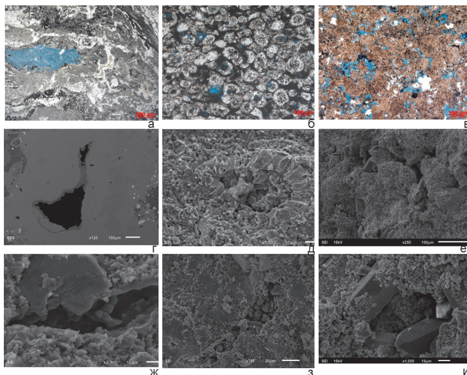
Рис. 5. Пустоты гидротермального выщелачивания в породах БАК. а, б, в – в шлифах; з-и – в образцах, исследованных методом растровой электронной микроскопии (РЭМ); а, з, ж – бактериально-водородные доломито-известняки; б, д, з – халцедон-кварцевые радиолариты; в, е, и – сфероагрегатные коллофановые фосфориты
