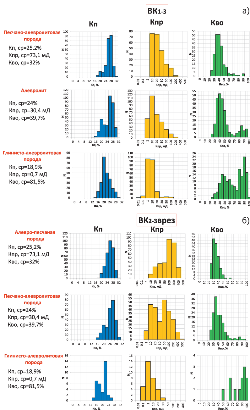
Рис. 1. Распределения петрофизических параметров по литофизическим типам пород пластов ВК 1-3 (а) и ВК 2-3 врез (б)
