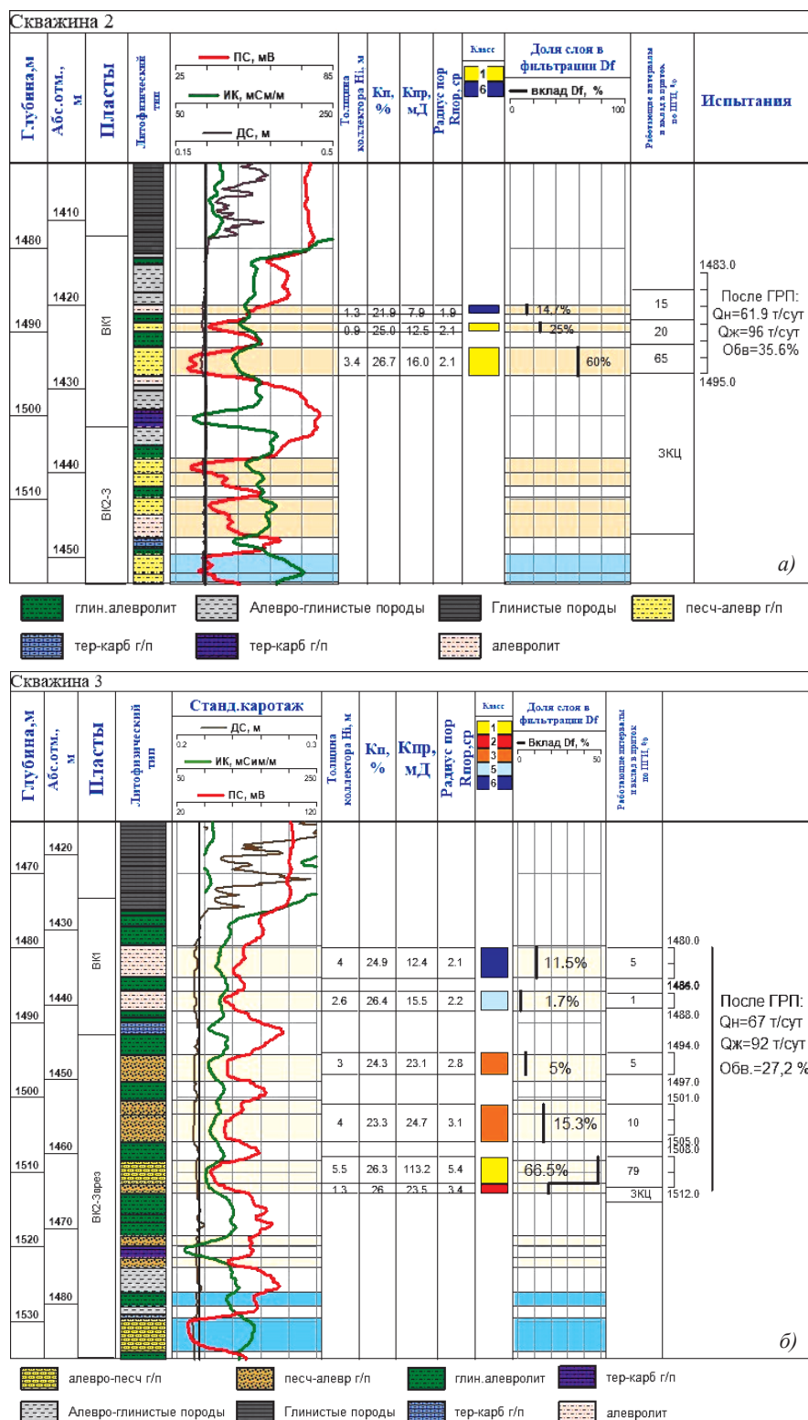
Рис. 8. Сопоставление расчетных и фактических результатов по ППИ по скважине 2 (а) и скважине 3 (б)
