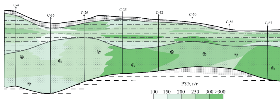
Рис. 9. Распределение РЗЭ в разрезе пласта диктионемовых сланцев и оболовых песчаников по профилю скважин C-4 – C-67. Условные обозначения см. на рис. 7. Масштаб горизонтальный 1:100 000, вертикальный для сланцев и песчаников 1:100, для надсланцевой толщи 1:1 000
