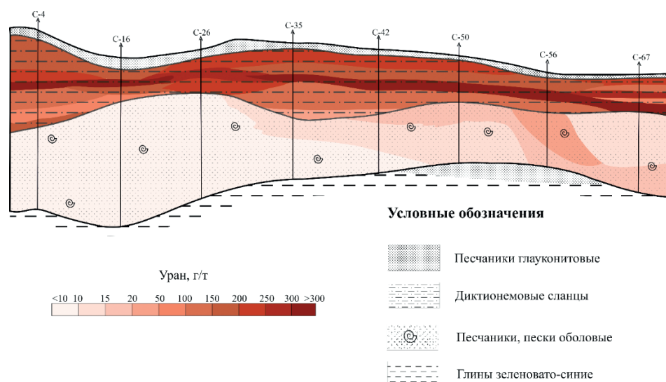
Рис. 6. Распределение урана в разрезе пласта диктионемовых сланцев и оболочковых песчаников по профилю скважин C-4 – C-67 по (Вялов и др., 2017). Масштаб горизонтальный 1:100 000, вертикальный для сланцев и песчаников 1:100, для надсланцевой толщи 1:1 000
