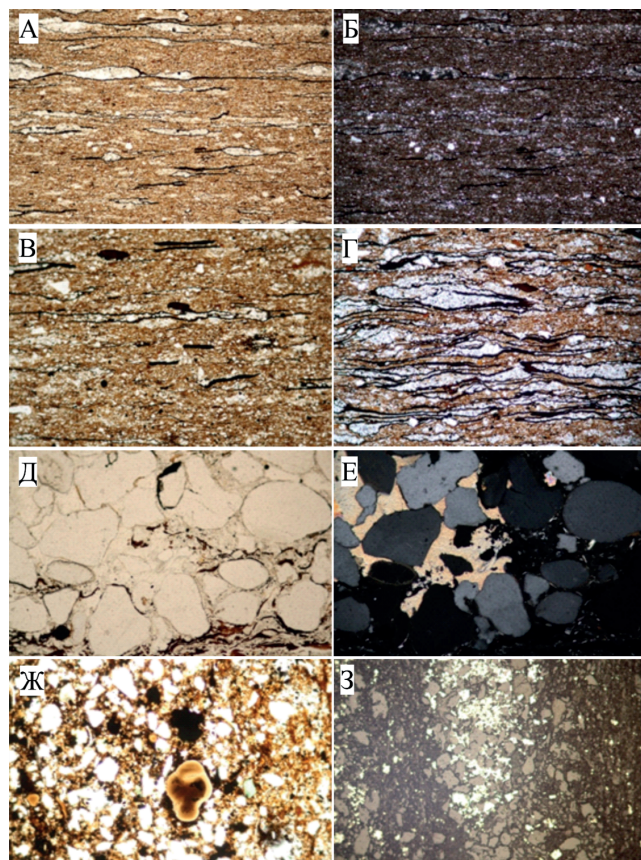
Рис. 4. Петрографический состав дикионемовых сланцев: А – коллоальгинит с глинистым веществом (николи ||, ув. \times 50 ); Б – то же (николи +, ув. \times 50 ); В – теки граптолитов в более глинистой части сланца (николи ||, ув. \times 100 ); Г – алевритовые гнезда (николи ||, ув. \times 200 ); Д – алевритовый прослой. Кварц, кальцит (николи ||, ув. \times 200 ); Е – то же (николи +, ув. \times 200 ); Ж – фосфатные конкреции (в центре, николи ||, ув. \times 200 ); З – вкрапленность сульфидов, глауконит (в центре, отраженный свет, ув. \times 200 )
