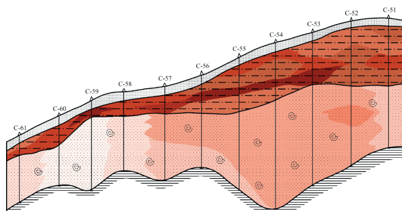
Рис. 7. Распределение урана в разрезе пласта диктионемовых сланцев и оболочковых песчаников по профилю скважин C-61 – C-51. Условные обозначения см. на рис. 6. Масштаб горизонтальный 1:100 000, вертикальный для сланцев и песчаников 1:100, для надсланцевой толщи 1:1 000
