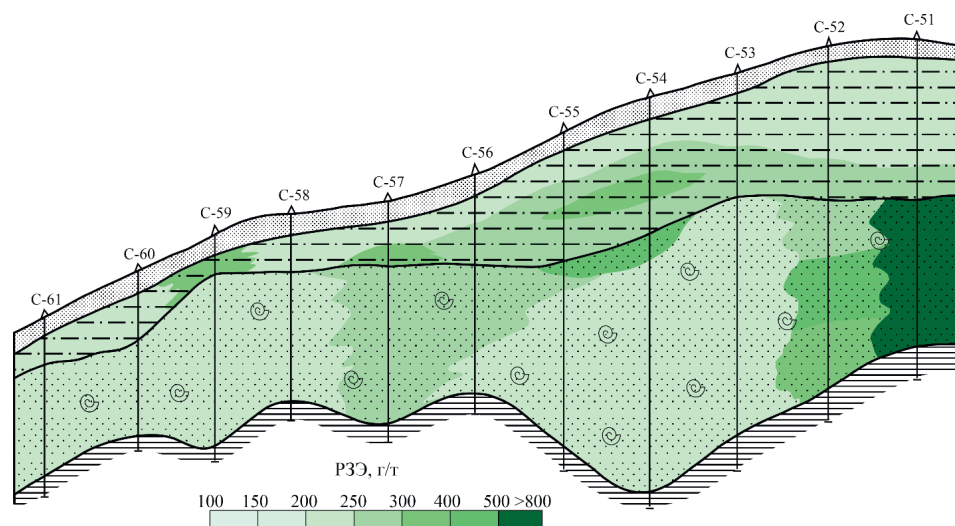
Рис. 10. Распределение РЗЭ в разрезе пласта диктионемовых сланцев и оболовых песчаников по профилю скважин C-61 – C-51. Масштаб горизонтальный 1:100 000, вертикальный для сланцев и песчаников 1:100, для надсланцевой толщи 1:1 000
