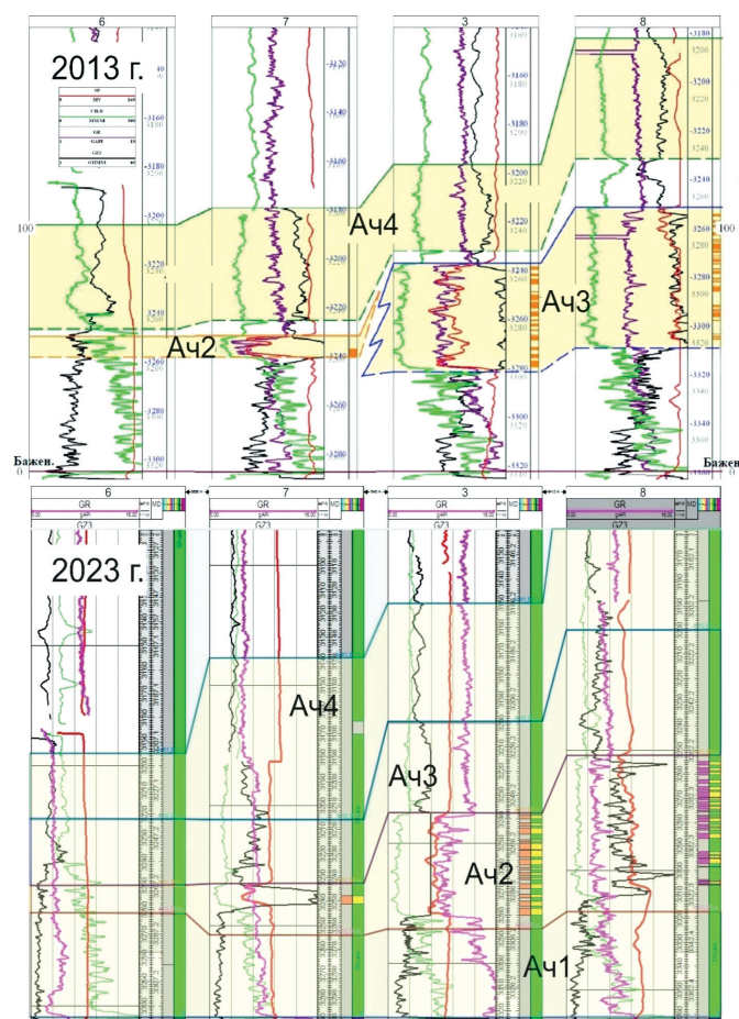
Рис. 3. Сопоставление скважинной корреляции пластов ачимовского интервала в пределах месторождения по данным 2013 года и результатам настоящих исследований
