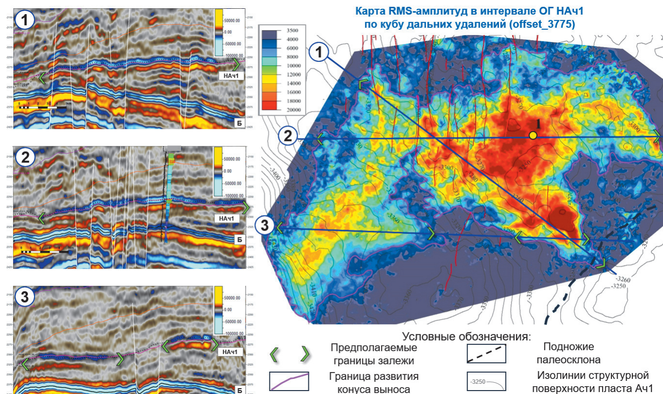
Рис. 5. Пример использования атрибута с куба дальних удалений при выделении объекта пласта Ач1 (объект выделен по граничному значению с графика)
