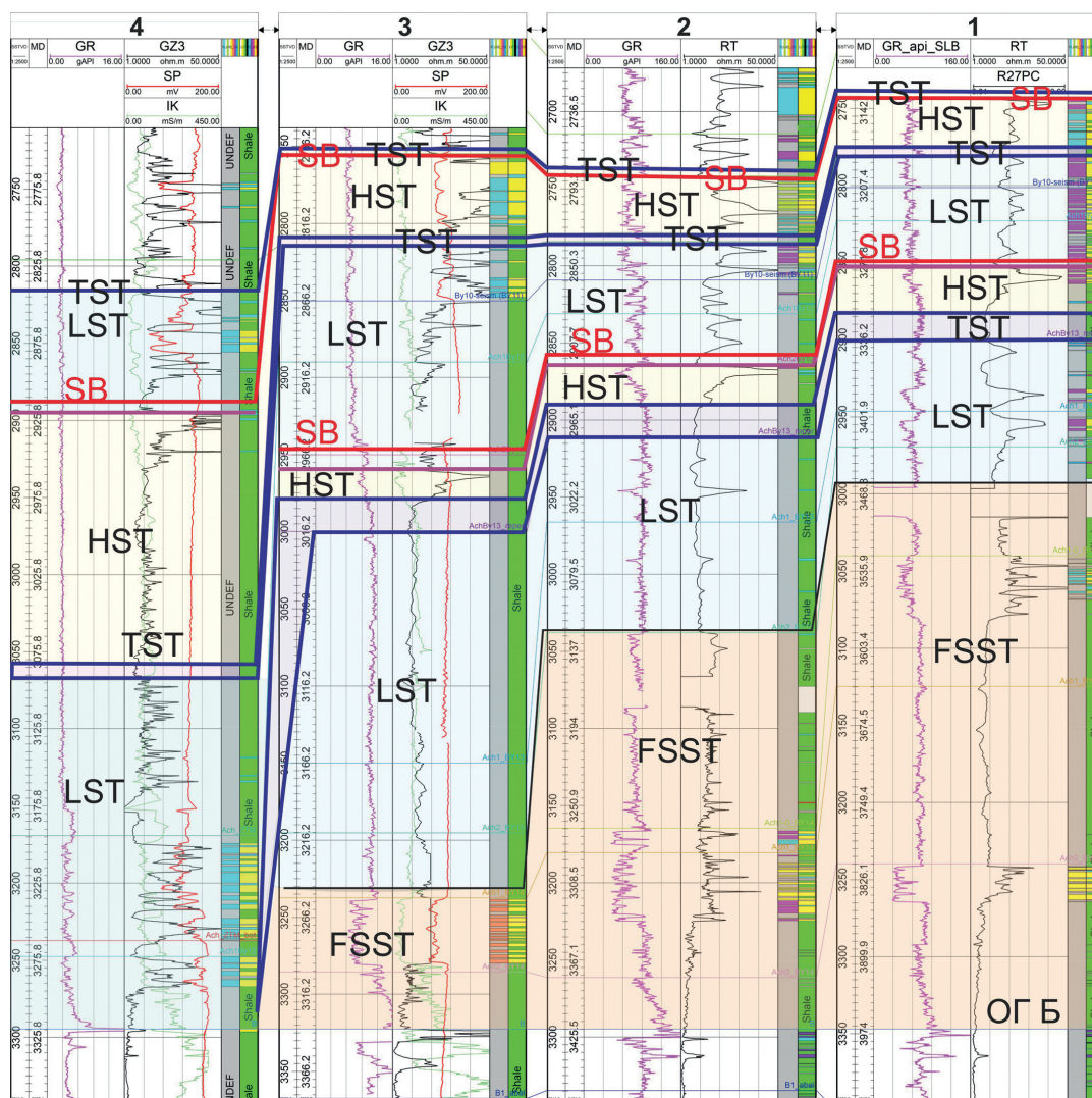
Рис. 2. Фрагмент схемы корреляции с указанием разбивок системных трактов в скважинах по линии временного разреза
