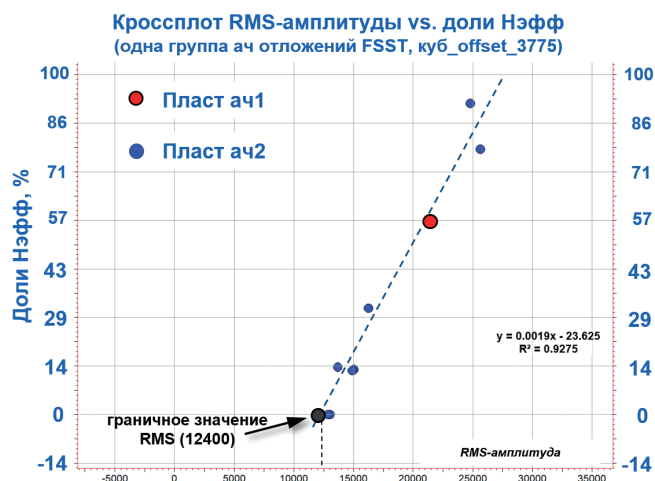
Рис. 4. График корреляции параметра доли эффективной толщины в скважинах со значениями атрибута в точках скважин для группы пластов Ач1, Ач2 системного тракта FSST
