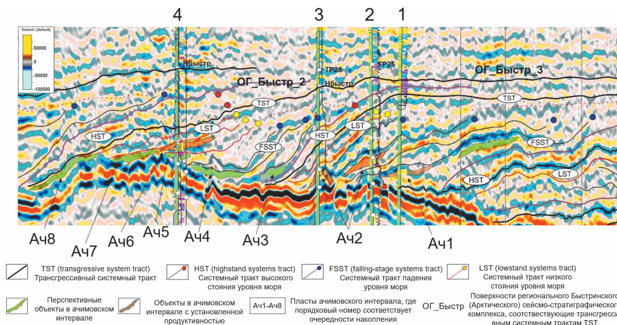
Рис. 1. Фрагмент временного разреза с нанесением данных интерпретации секвенс-стратиграфического анализа и материалов скважин
