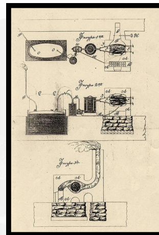
Схема термолампы Соболевского, (дело №533 в государственном историческом архиве), достойная украсить марочный блок.
