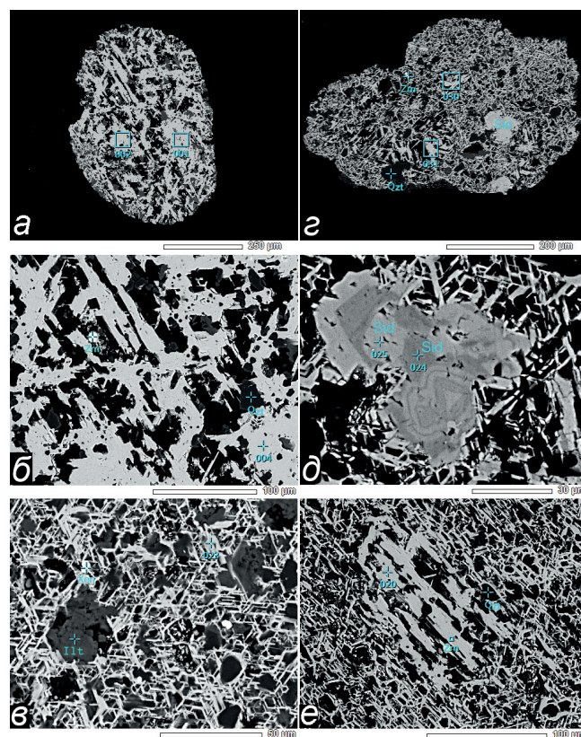
Рис. 7. Изображения (режим BSE) зерен рутилового лейкоксена. а – проба МПЛ-2, з – проба ПЖ-45 (Пижемское месторождение) и их увеличенные фрагменты (б, в, д, е), д – включения зональных кристаллов сидерита и номера их анализов. Рамки – места анализов сканированием по площади и расположение зонда рамановской спектроскопии, крест – точечные анализы и их номера по спектрам ЭДС: Qzt – кварц, Zrn – циркон, Illt – иллит, Sid – сидерит, Xep – ксенотим
