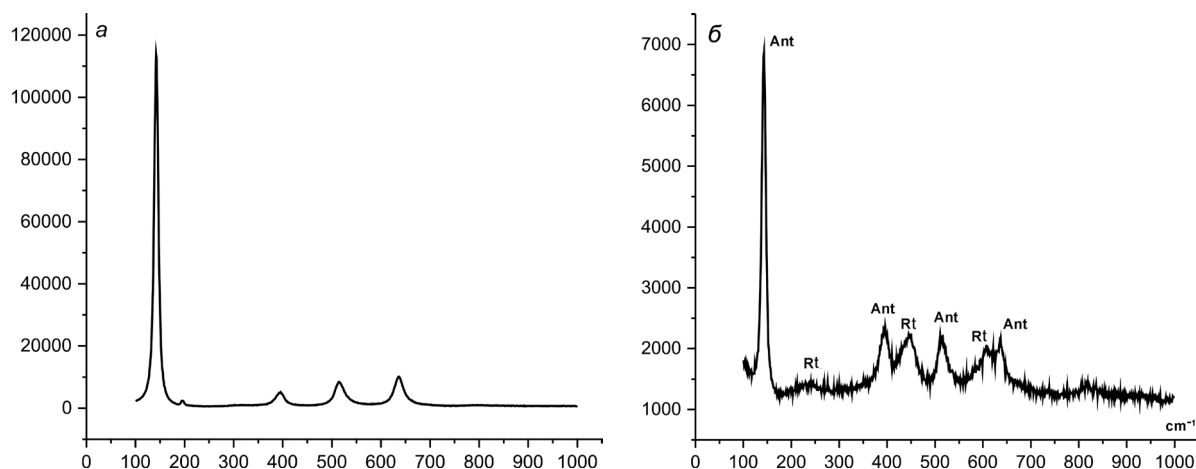
Рис. 4. Рамановские спектры: а – кристалла анатаза (15d1) из Ярегского месторождения с характерными пиками: 145, 195, 395, 520, 635 \text{см}^{-1} ; б – смеси выделений рутила (Rt) и анатаза (Ant) в зерне № 17 из Ярегского месторождения (см. рис. 1) с характерными пиками: анатаз – 145, 395, 520, 635 \text{см}^{-1} , рутил – 240, 450, 610 \text{см}^{-1}
