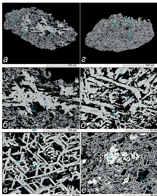
Рис. 6. Изображения (режим BSE) зерен лейкоксена (а – проба МЯР, Ярегское месторождение; з – проба МПЛ-1, Пижемское месторождение) и их увеличенных фрагментов (б, в, д, е). Рамки – места анализов сканированием по площади и расположение зонда рамановской спектроскопии, крест – точечные анализы и их номера. Белые крупные пятна – псевдуртил, Qzt – качественные определения кварца по спектру ЭДС. Номера анализов совпадают с номерами в таблицах химических анализов
