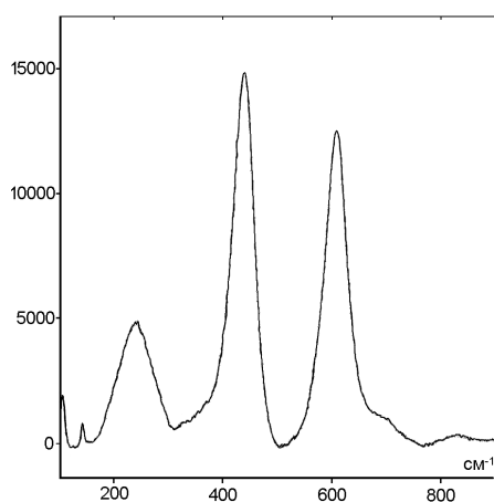
Рис. 5. Типичный рамановский спектр рутила. Перекристаллизованные кристаллы рутила размером 50–150 мкм из зерна пижемского лейкоксена с пиками – 240, 450, 610 \text{см}^{-1}
