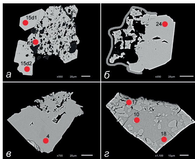
Рис. 2. Изображения (режим BSE) типичных мелких кристаллов анатаза из Ярегского месторождения: а, б – нарастание новообразованных кристаллов анатаза на зерна анатазового лейкоксена (15 и 24), черные включения – кварц; в – отдельный кристалл анатаза (4); г – фрагмент сростка (17) рутила и анатаза (белый). Красные точки – расположение зонда рамановской спектроскопии и номера спектров
