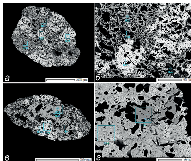
Рис. 8. Изображения (режим BSE) двух зерен (а, в) рутилового лейкоксена в сростании с фрагментами псевдуртила (белое) проба МПИ-2 и их увеличенных фрагментов (б, з), Пижемское месторождение. Рамки – места микрозондовых анализов сканированием по площади, кресты – точечные анализы и их номера
