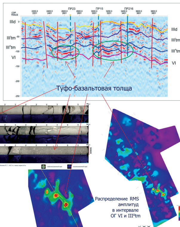
Рис. 5. Выделение туфо-базальтовой толщи в интервалах разреза Нижнечутинского месторождения
