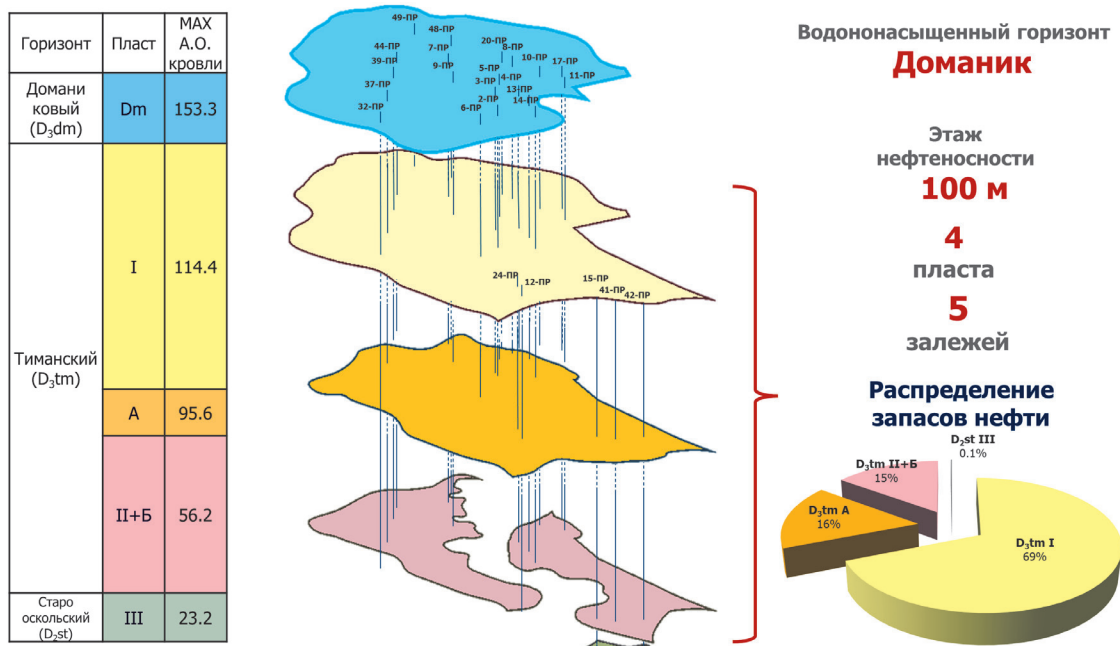
Рис. 1. Продуктивные отложения Нижнечутинского месторождения
