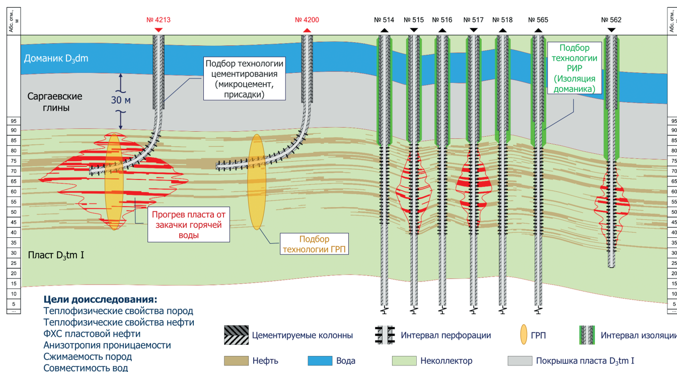
Рис. 7. Апробация технологических решений для эффективной разработки продуктивных отложений Нижнечутинского месторождения
