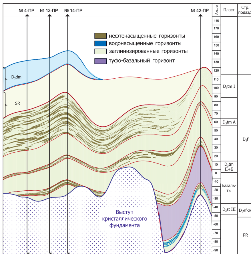
Рис. 2. Геологический разрез Нижнечутинского месторождения
