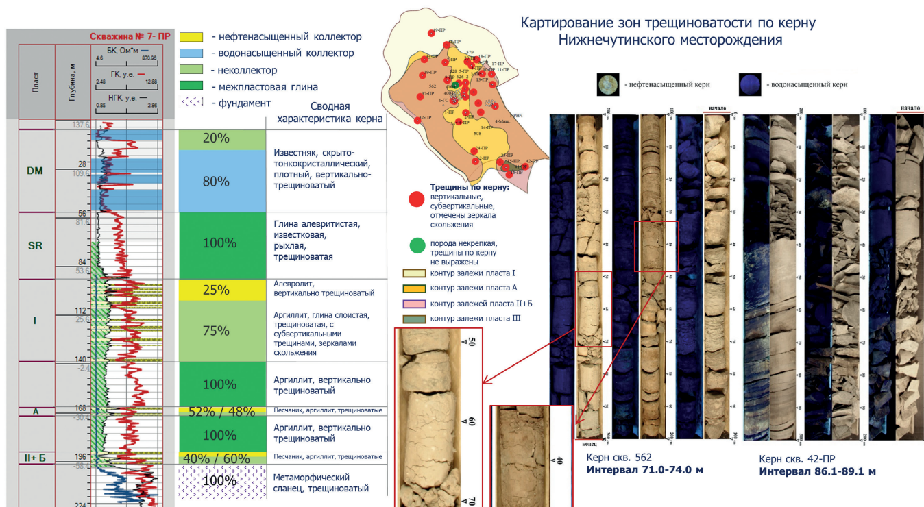
Рис. 3. Характеристика слагаемых продуктивных горизонты пород
