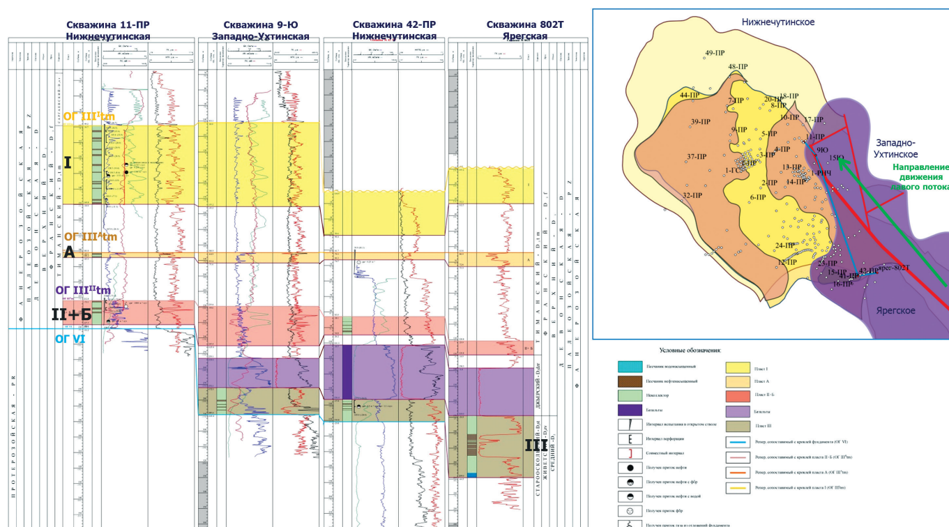
Рис. 4. Прослеживание эффузивных пород в разрезе Нижнечутинского месторождения
