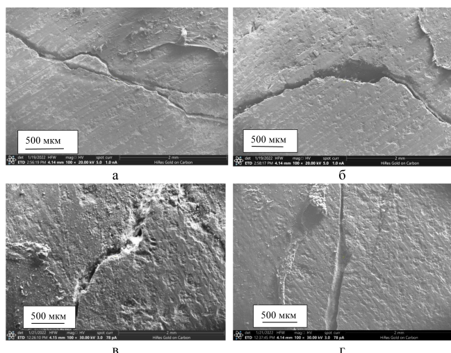
Рис. 5. Типичные трещины в образцах керна для литотипа 2 (а, б) и литотипа 3 (в, г), образованные после создания напряженного состояния пород
