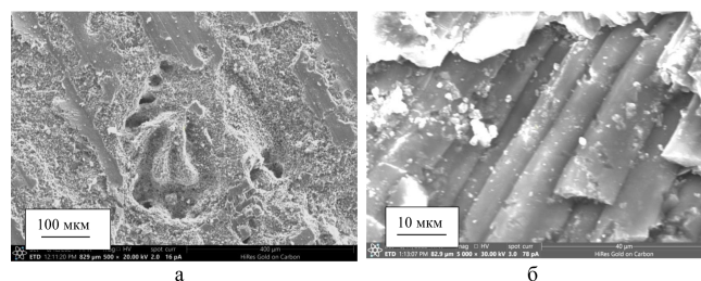
Рис. 3. Типичные признаки генетических типов известняка: а – фораминиферовый (литотип 2), б – водорослевый (литотип 3)
