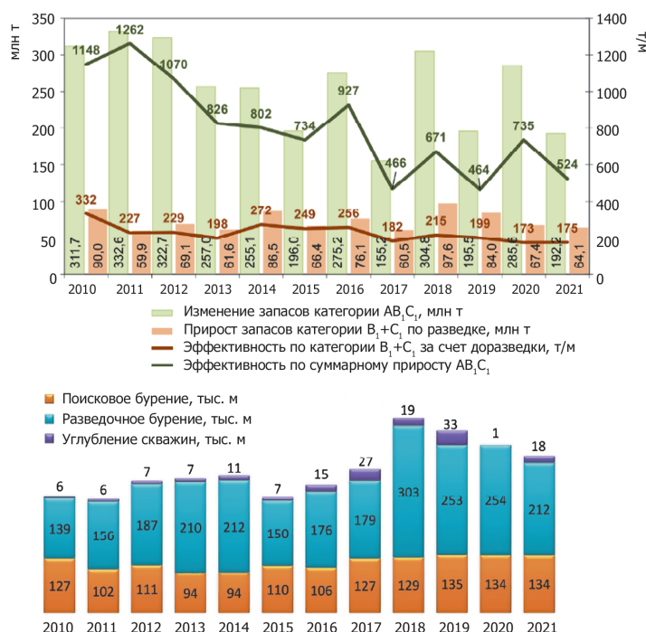
Рис. 4. Показатели эффективности ГРП за период 2010–2021 гг. для территории ХМАО – Югра (по данным Ежегодного аналитического обзора «Недропользование в Ханты-Мансийском автономном округе – Югре в 2021 году», 2022)
