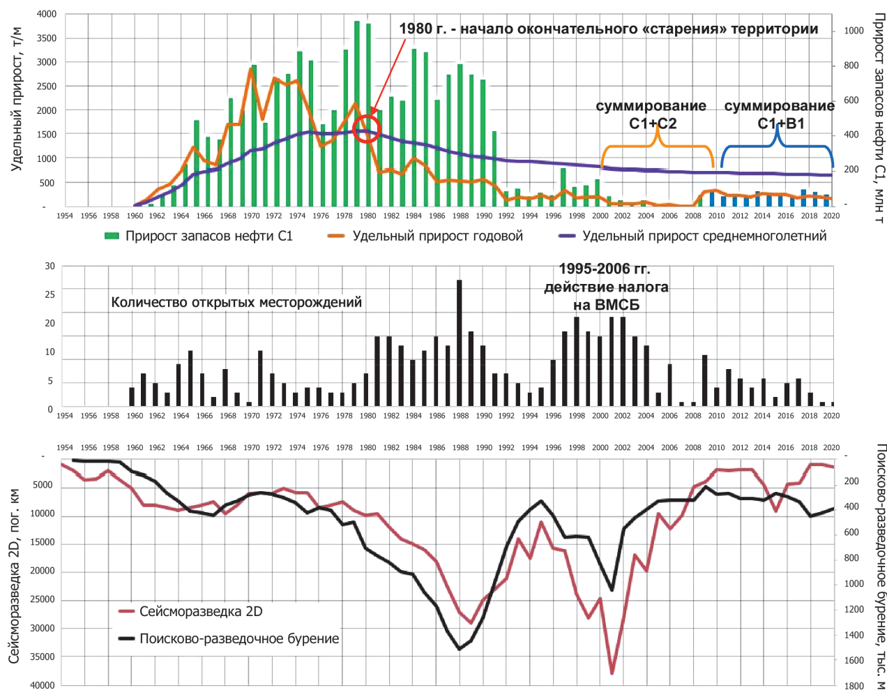
Рис. 3. Ретроспективный анализ эффективности ГРП для территории Широ́тного Приобья (ХМАО – Югра)
