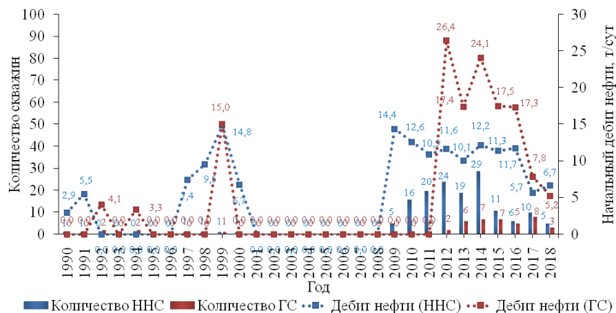
Рис. 3. Динамика ввода скважин и их начальная технологическая эффективность в разрезе «Южной» группы месторождений
