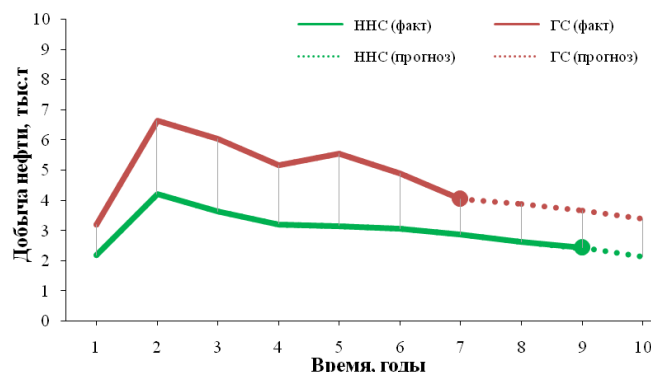
Рис. 5. Динамика работы скважин различного профиля (объекты группы «Ю₁»)
