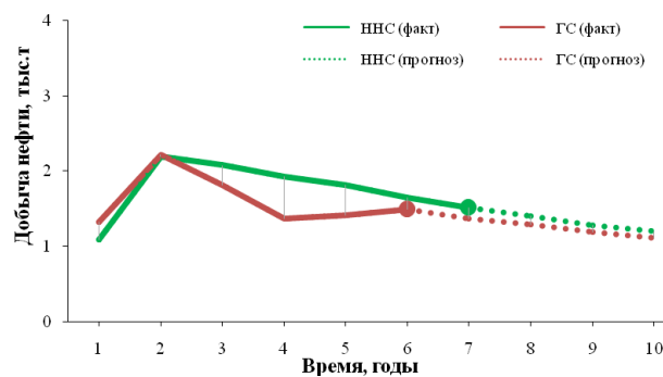
Рис. 6. Динамика работы скважин различного профиля (объекты группы «Ю₂»)
